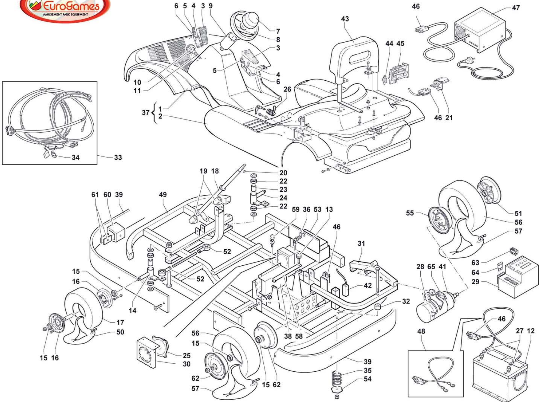
Mod. MINI GO-KART - 12V Cod. 6900
